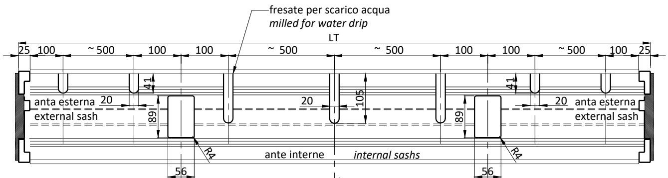
Fori di fissaggio PR2983-PR2984 al PR1195 Fixing holes PR2983-PR2984 to PR1195
