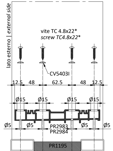
Fori di fissaggio Anchoring holes
